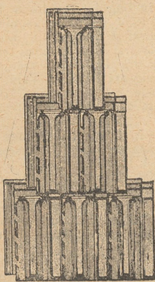
Fabric. de Nagyikinda. Țigle de siguranță pentru acoperiș, patentate, sistem Bohn, Nr. 272.
