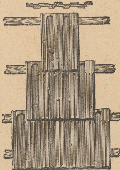
Fabricat de Zsombolya Țigle de siguranță pentru acoperiș patentate Nr. 253.
