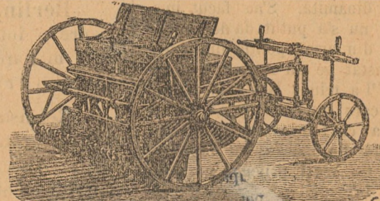
Mașină ușoară de sămănat „Königs Drill”.
