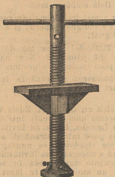
Fus pentru piua de ulei.
