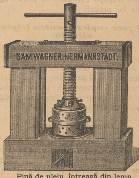
Piuă de ulei, întreagă din lemn.
