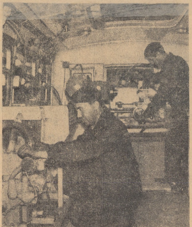
Atelierul mecanic mobil, produs de uzina Automecanica Mediaș, înzestrat cu strung, grup electogen, polizor, motopompă, aparat de sudură etc., este destinat lucrărilor de reparații, pe șantier, în campanii agricole sau exploatare forestiere.
