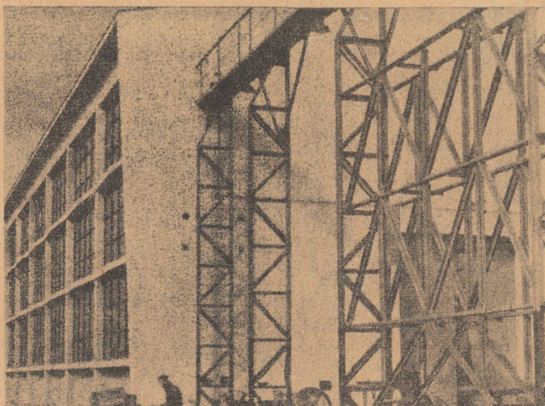
Hala reparații gateră de la I.R.U.M. Sibiu
