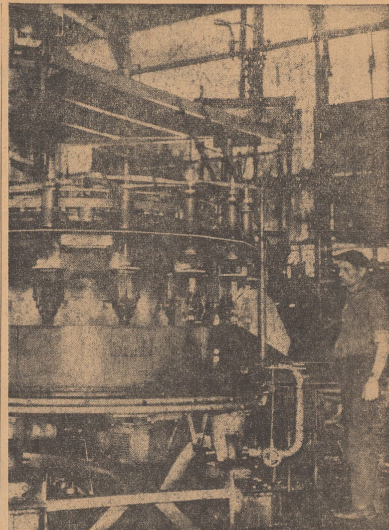
Muncitorul care supraveghează mașina de suflat prin rotire a articolelor din sticlă, produse de „Vitrometan”. Mediaș, are doar cîteva atribuți: menținerea la nivel constant a temperaturii, a presiunii de aer pentru răcire și a nivelului de sticlă fluidă.
