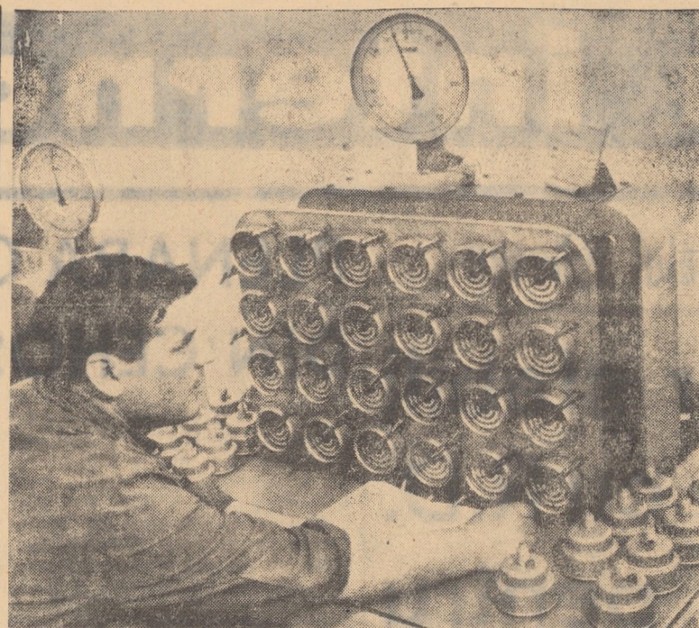
Uzina „Balanta”, Sibiu. Maistrul Romulus Vasu verificînd la bancul de probă un nou lot de viteze.
