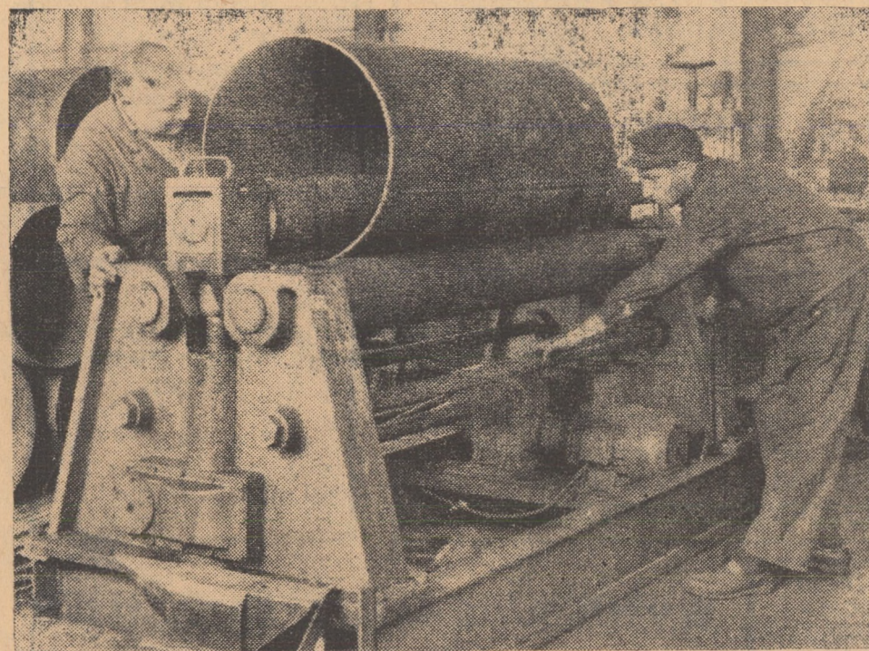
Calandru pentru îndoit tablă, re- alizat prin mică mecanizare la u- zina „Automeca- nica” din Sibiu
