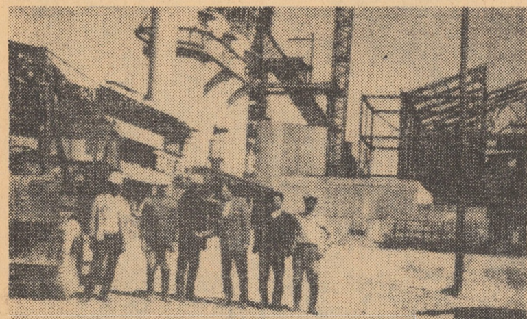
ALGERIA — În orașul Annaba se construiește un mare combinat metalurgic. Prima parte a combinatului va produce anual 350.000 tone de oțel. Combinatul va începe să producă în anul 1969. În fotografie: Unul din sectoarele de construcție a combinatului.
