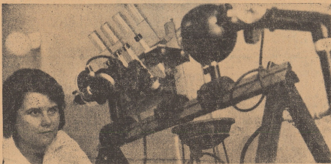
La I.L.S. „Amylon” — Sibiu, etalonul de culoare a glucozei lichide se stabilește cu ajutorul fotocolorimetruului. În fotografie: ing. Nadia Filip, efectuînd această probă
