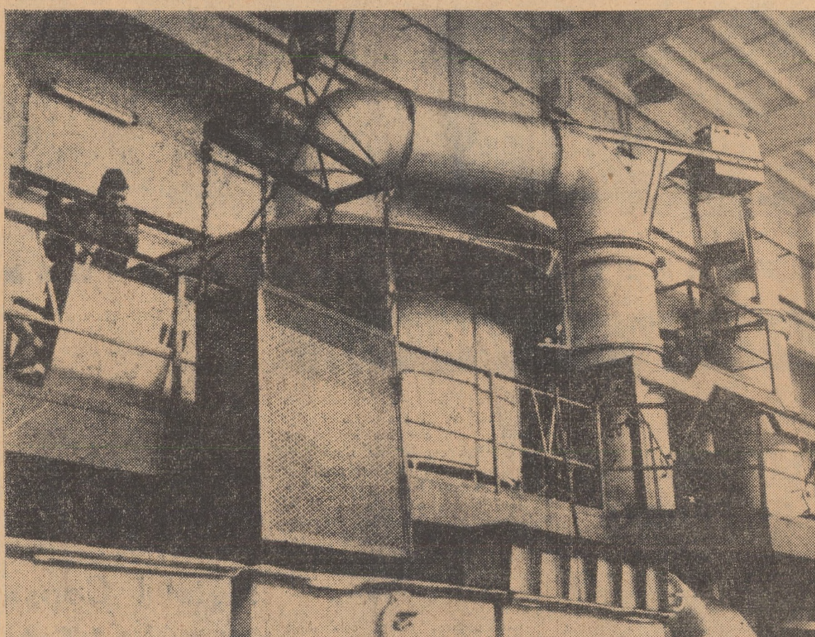
Faza de decapare a barelor susținătoare ale catodilor, din procesul de topire și rafinare a plumbului de la U.C.M. Copsa Mică
