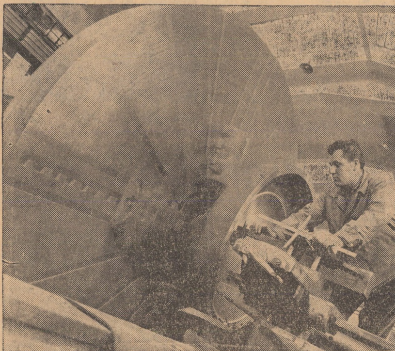
Suporturile pentru lagăr steric, produse de uzina Independența, „Sibiu”, necesare granulațoarelor giratorice Ø 1250, folosite în industria minieră, sînt prelucrate la o mașină frontală de strunjit, deservită de Gheorghe Pilași, fruntaș în întrecerea socialistă
