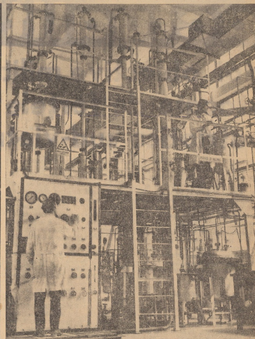
Instalația pentru studiul valorificării acetonitrilului din secția „sinteză organică a Institutului „Chimgaz” din Mediaș
