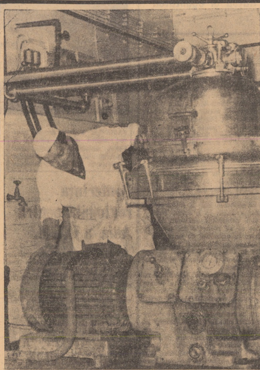
Printre utilajele moderne, cu care a fost înzestrată fabrica „Berea Sibiului”, se numără și separatorul centrifugal, folosit la separarea trubului de mustul de bere
