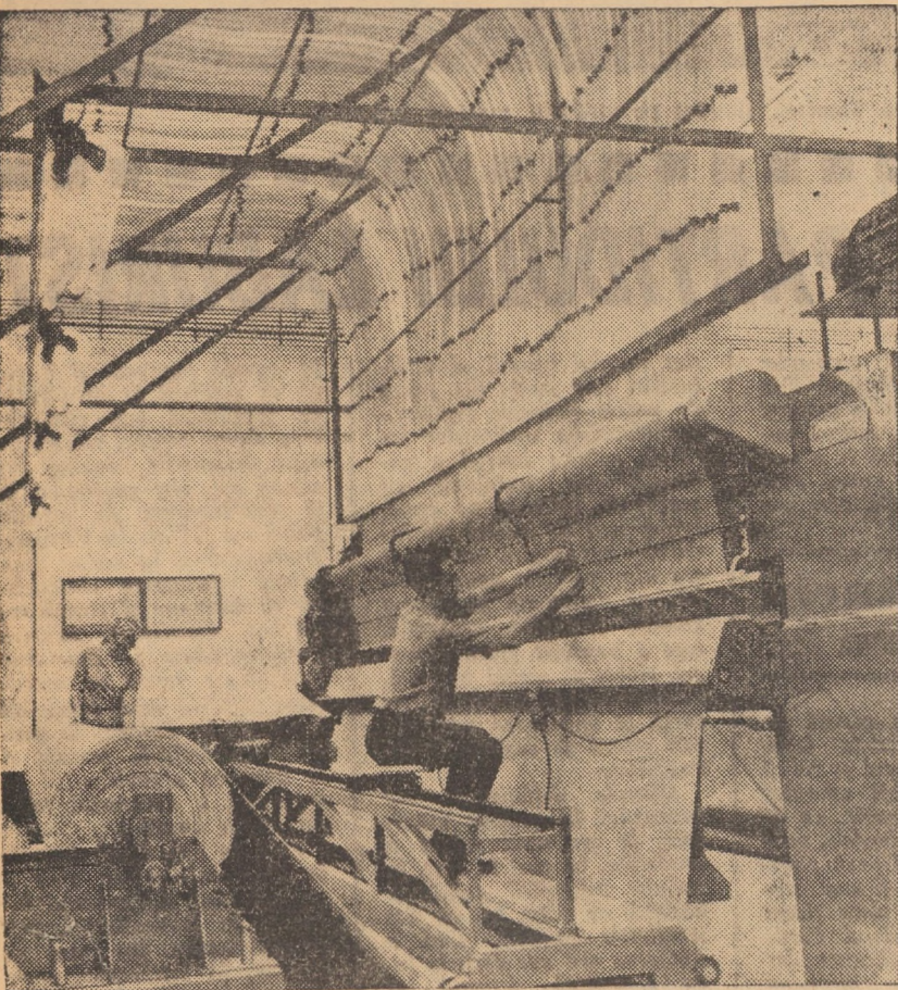
În secția covor pusat a Uzinelor textile Cisnădie, noua mașină „Tufting”, utilaj modern de mare productivitate, recent pusă în funcțiune, realizează în 8 ore cca. 600 metri pătrați covor, avînd o lățime de 5 metri
