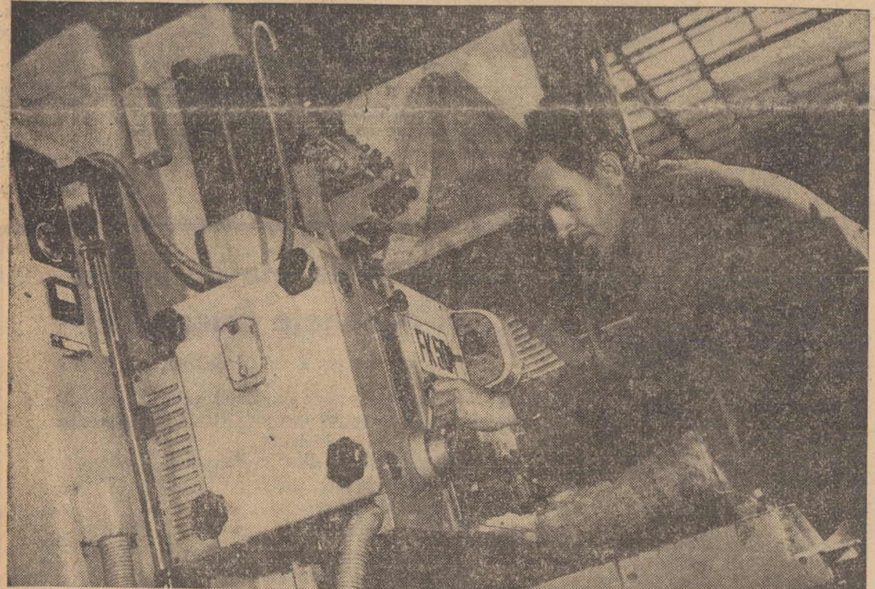
Uzina „Automecanică”, Sibiu. În secția școlară, matricele și alte dispozitive cu profil complicat, necesare S.D.V.-urilor, constituind echipamentul tehnologic al produselor executate în uzină, sînt prelucrate cu ajutorul unei mașini de frezat prin copiere cu comandă electronică prin impulsuri deservită de comunistul Eduard Glatzer
