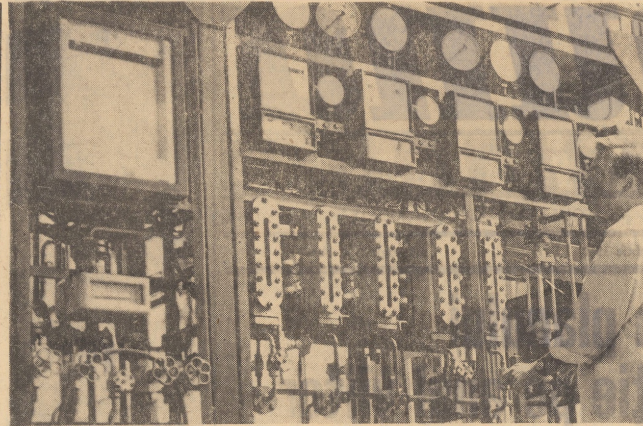
Secția sinteze organice a Institutului „Chimigaz” din Mediaș: instalația pentru sinteza etanolaminelor. Foto: FRED NUSS
