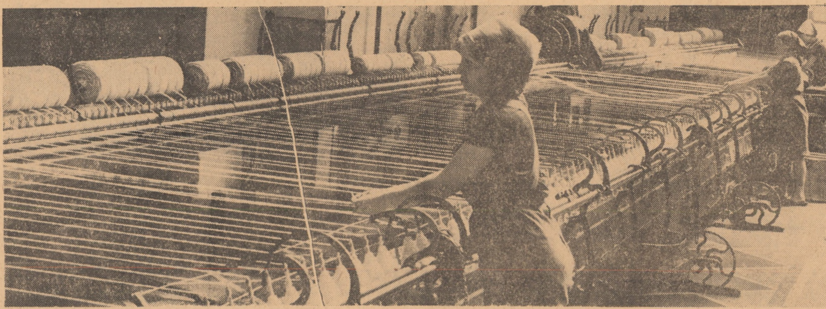
Fabrica „Dumbrava” Sibiu. Se pregătesc firele necesare secției de țesătorie a covoarelor
