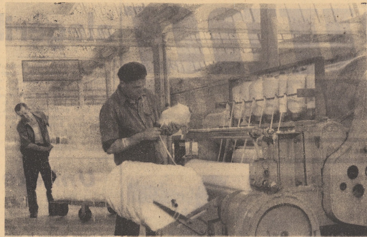
Uzina „Trnava” Mediaș, secția bătăj. Una din mașinile la care se execută operațiile de destrămare, eliminarea impurităților și depunerea masei de fibre
