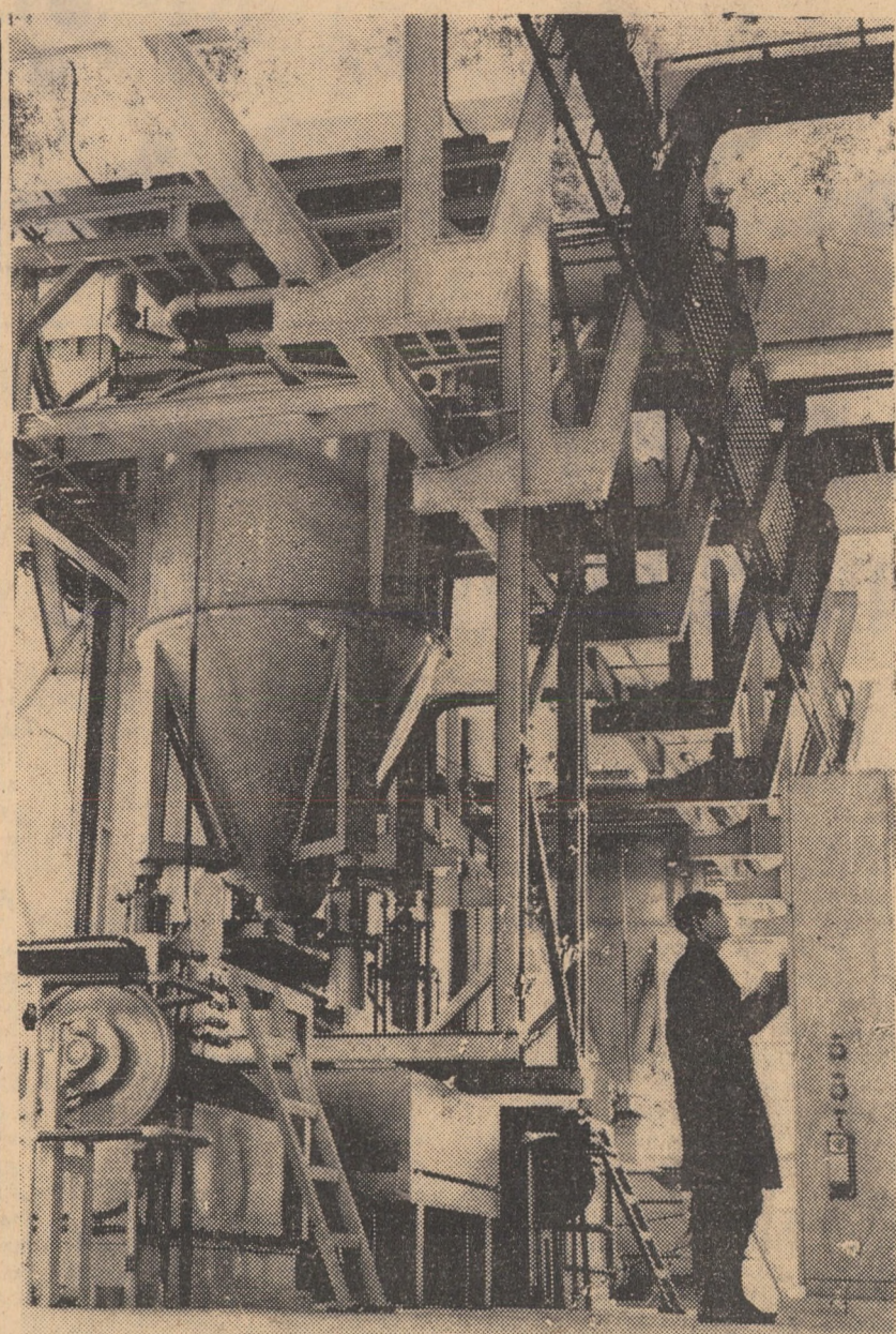
Instalația de omogenizare a materiilor prime în cadrul fluxului de fabricare a fritei de la uzina „Email roșu”
