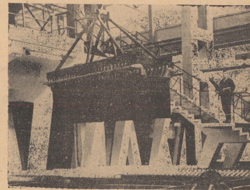
Aspect din secția electroliză a plumbului de la U.C.M. Copșa Mică
