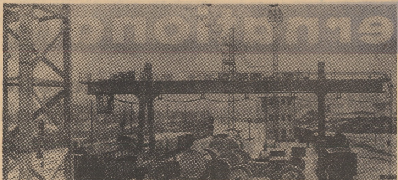
Rampa de încărcare și descărcare a mărfurilor din gara Sibiu dispune de macara portală cu ajutorul căreia sînt manipulate mărfurile de mare greutate
