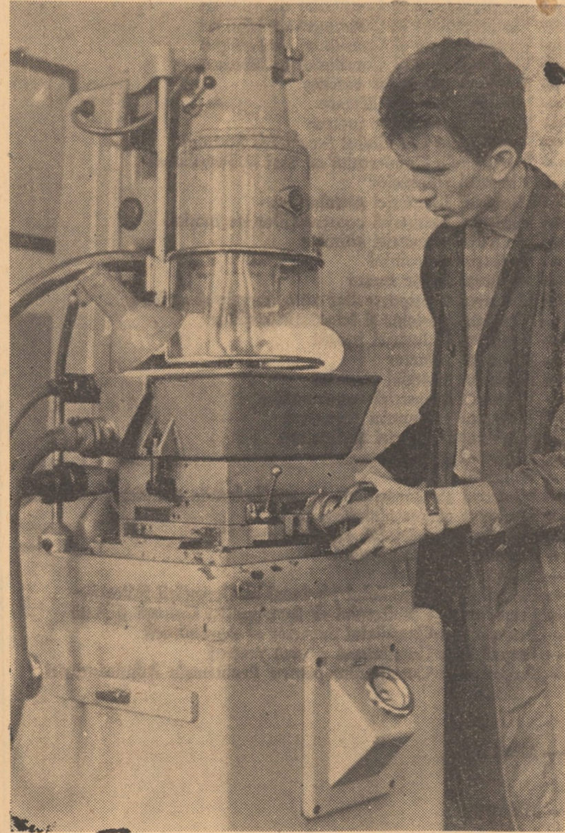
Matrițele cu profile speciale, necesare la procesul de injectat al masei plastice pentru produsele fabricii „Flamura roșie” Sibiu...
