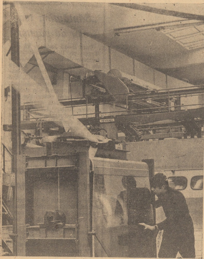
În secția albire a fabricii „Tirnavă” Medias Foto: FRED NUSS
