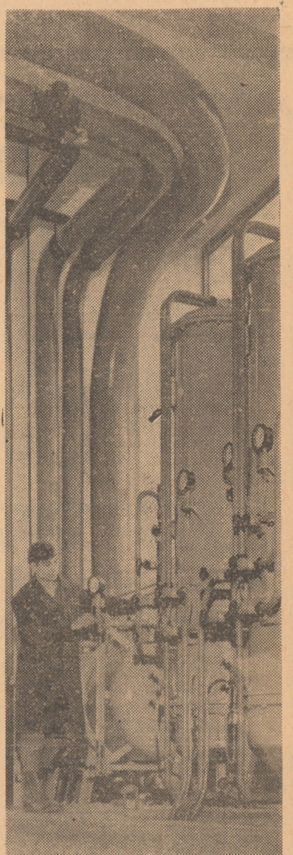
Stația de demineralizare a apei, necesare procesului de fabricare a emailurilor la uzina „Emailul roșu” Mediaș
