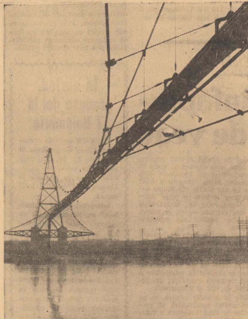
O traversare aeriană a unei conducte de transport gaze peste unul din rîurile mari ale țării
