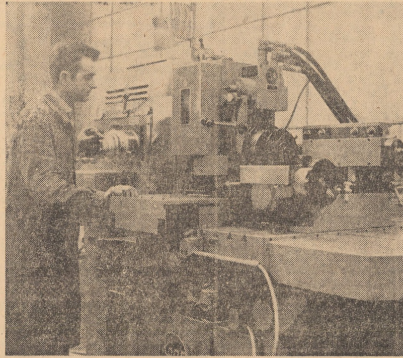
Mașina de rectificat came prin copiere. Rectificator: Gheorghe Bogorin, de la uzina „Balanța” Sibiu. Foto: VICTOR PELGER
