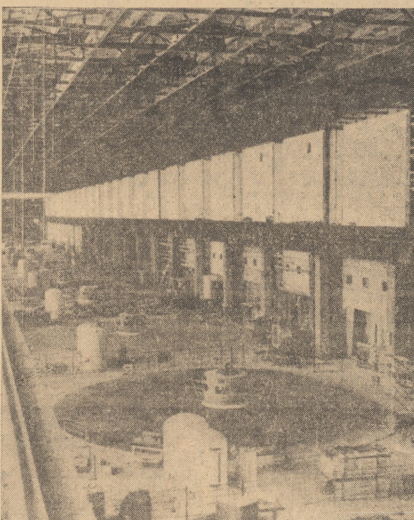
U.R.S.S. La hidrocentrala din Krasnoiarșk a intrat în construcție cel de-al 9-lea agregat cu o putere de 0,5 mil. kW. Prin intrarea în funcțiune a ultimului agregat (al 10-lea) hidrocentrala, deja cea mai puternică din lume, va furniza 5 mil. kW. În foto: Vedere din sala mașinilor la hidrocentrala din Krasnoiarșk
