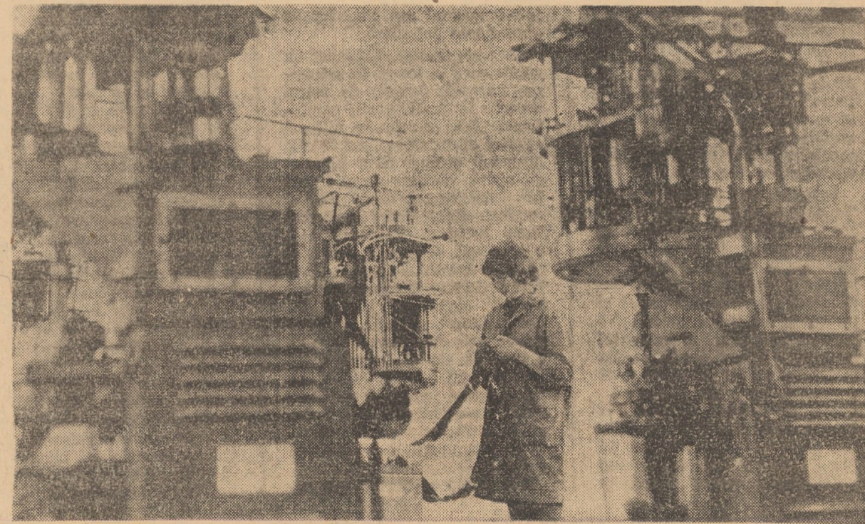
Mașini moderne de tricatat, de mare randament, asigură astăzi o producție de ciorapi de bună calitate. Cadru din secția dublu cilindru a Fabricii de tricotație Agnita, a Combinatului de ciorapi și tricotație Sibiu
