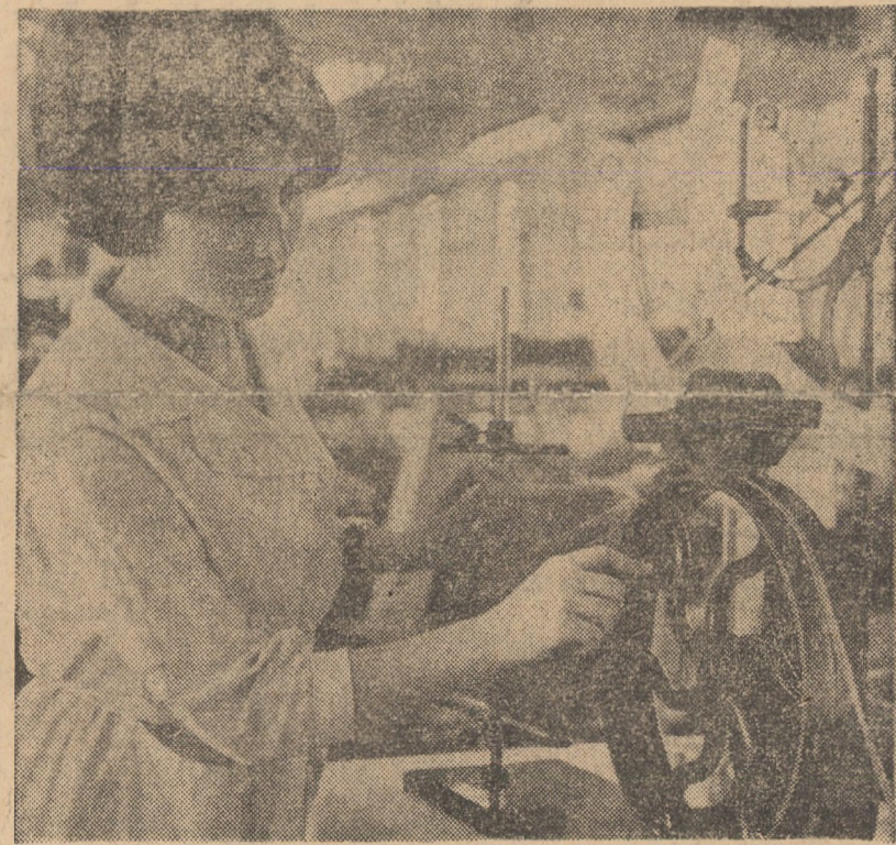
La secția preparării filaturii a fabricii „Libertatea” din Sibiu, sint efectuate probe de laborator pentru determinarea unor eventuale neuniformități ale materialului. În fotografie: laboranta Emilia Bozdoc în timpul lucrului
