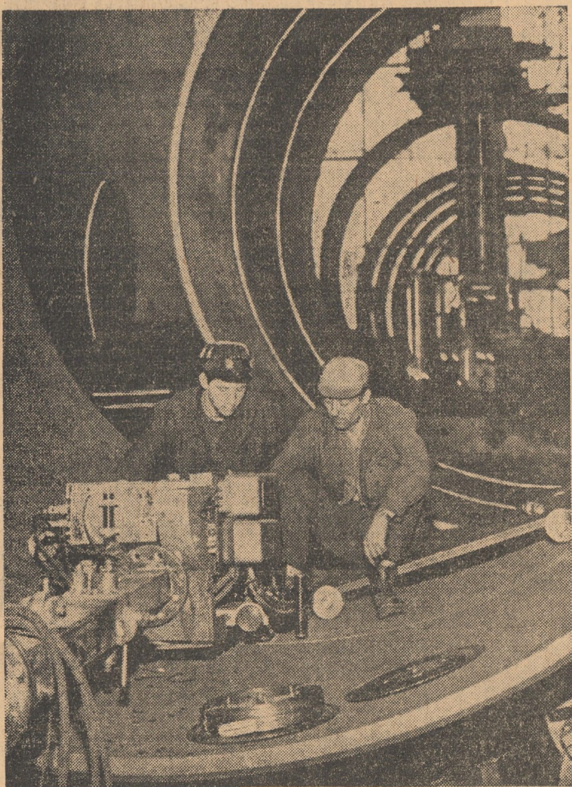
Asamblarea virolorelor, produse de cazangeria uzinei „Independența” Sibiu, se realizează cu ajutorul procedurii de sudură electrică automată, procedeu care asigură o productivitate a muncii ridicată și o calitate net superioară a sudurii. În fotografie: sudorii Traian Covașe și Liviu Sărățean în timpul lucrului
