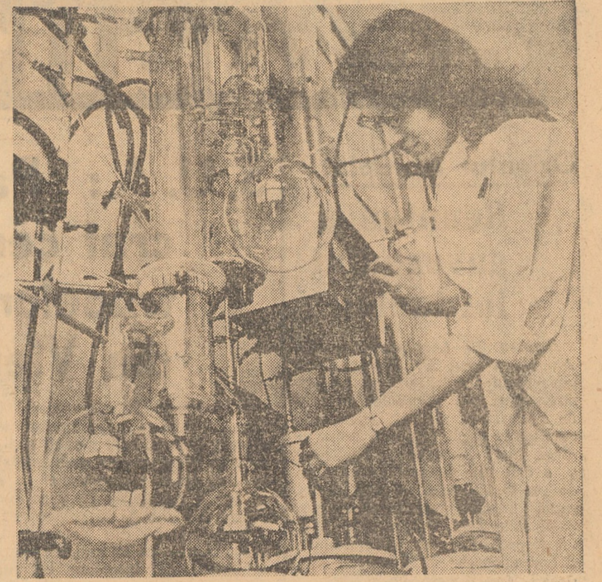
Institutul „Chimigaz” Mediaș. Aparat de distilare moleculară, folosit la distilarea substanțelor organice termo-labile
