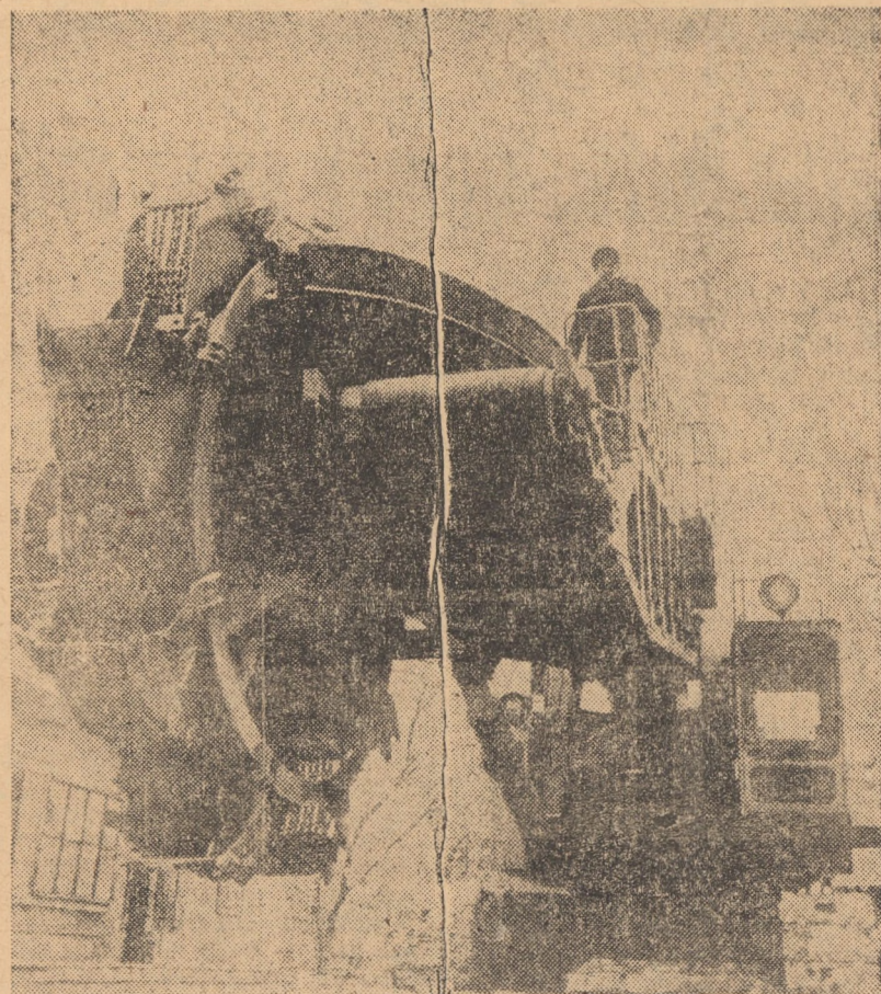
U.R.S.S. Uzina de excavatoare din Voronej produce excavatoare universale pe șenile cu o capacitate de încărcare de 1,25 și 2,5 m.c. cu transmisie Diesel și electrică. La aceste excavatoare se pot monta și macarale ce pot ridica o greutate de 20 și 60 de tone. Cea mai bună realizare a constructorilor uzinei este excavatorul rotativ R-100, care poate înlocui munca a 500 de săpători
