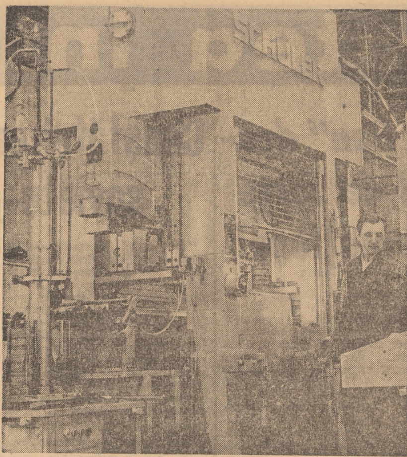
Uzina „Emailul roșu” Medias. Prese cu transfer de 60 tone, la care se execută accesorii pentru vase, efectuind 6 operații simultane
