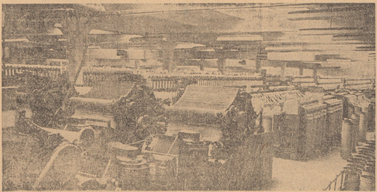
Aspect din secția preparăția filaturii de bumbac „11 Iunie” din cadrul Combinatului textil Cisnădie
