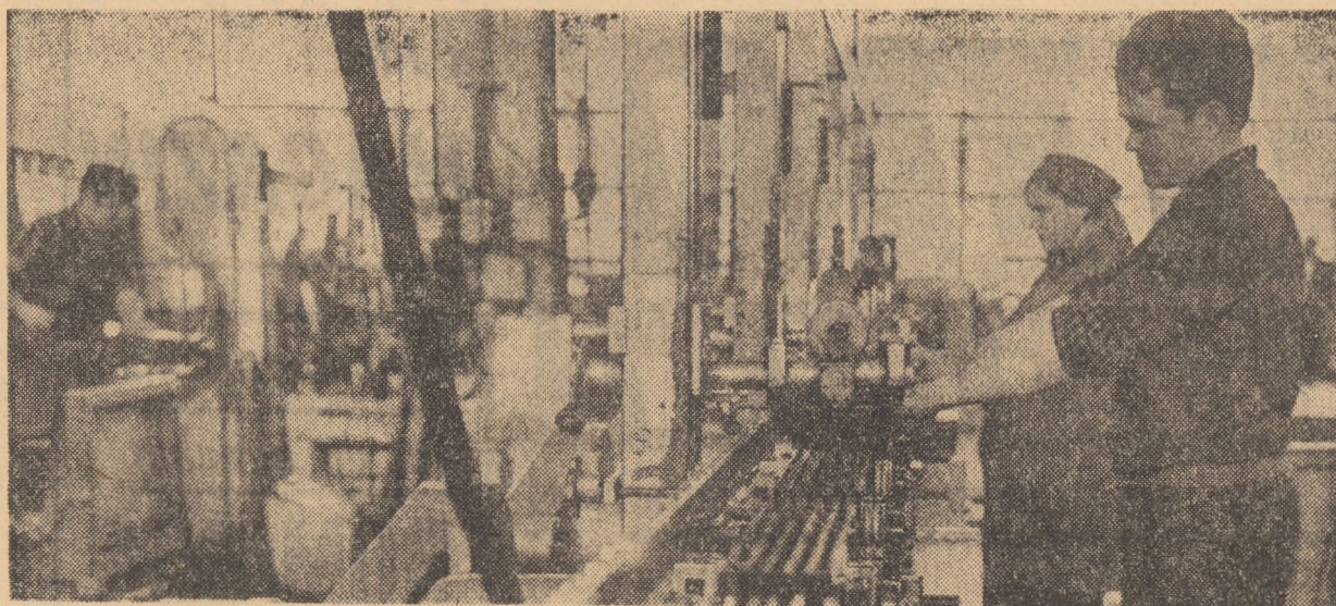
Fabrica de geamuri Mediaș. În secția prelucrare, unul din utilajele asigură șlefuirea canturilor la geamuri plane de diferite dimensiuni. La această mașină se execută lunar, șlefuiți de 70 000 metri liniari
