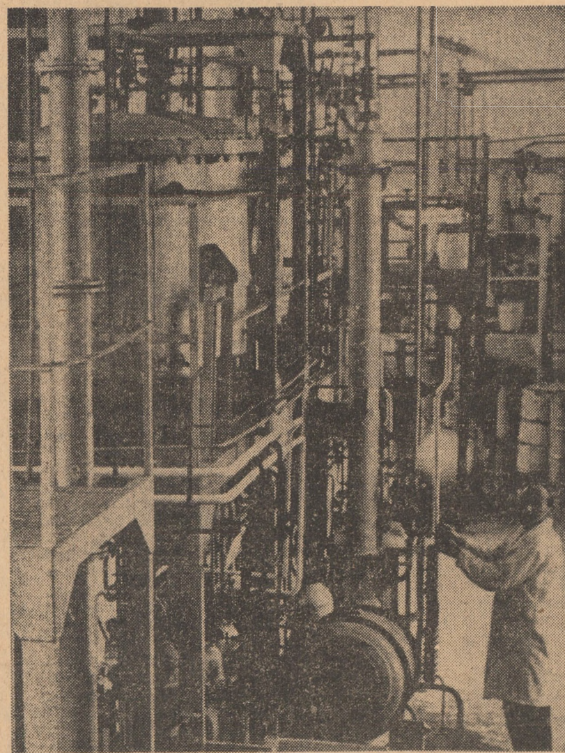
Instalație pilot, la institutul „Chimigaz” Mediaș
