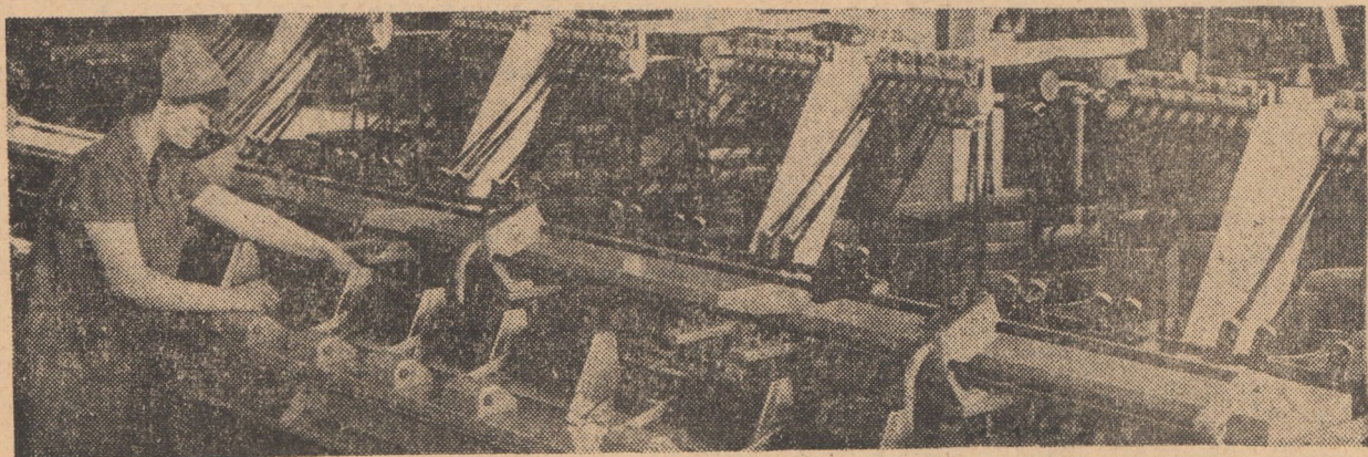
Laminor de mare întindere cu 32 câni. Fabrica „Libertatea” a Combinatului textil Sibiu
