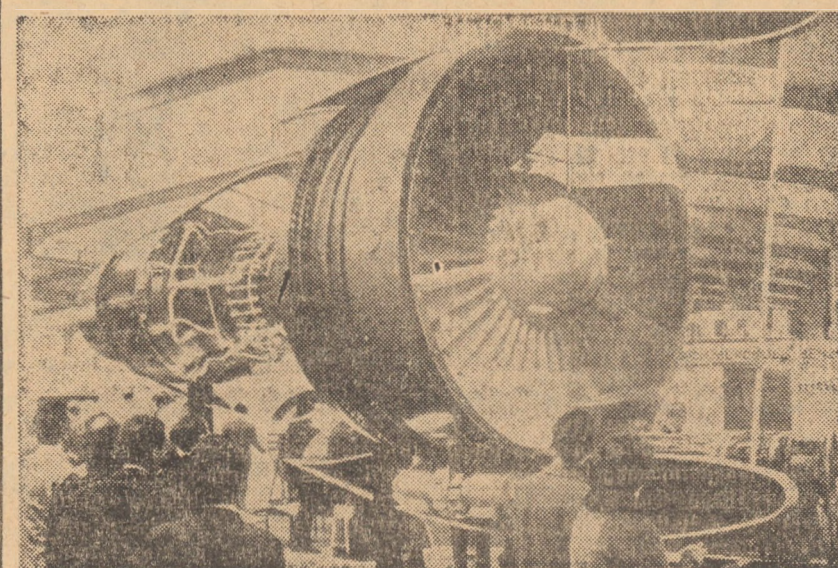
R.F. a GERMANIEI. La Expoziția Internațională aeronautică de la Hanovra, printre altele expozate, a putut fi văzut cel mai mare motor turbinoractor din lume, care cîntărește 3,5 tone. Motorul, construit la „Motoren Turbinen Union” din München, urmează să fie folosit la „Aerobuzul A-300 b”
