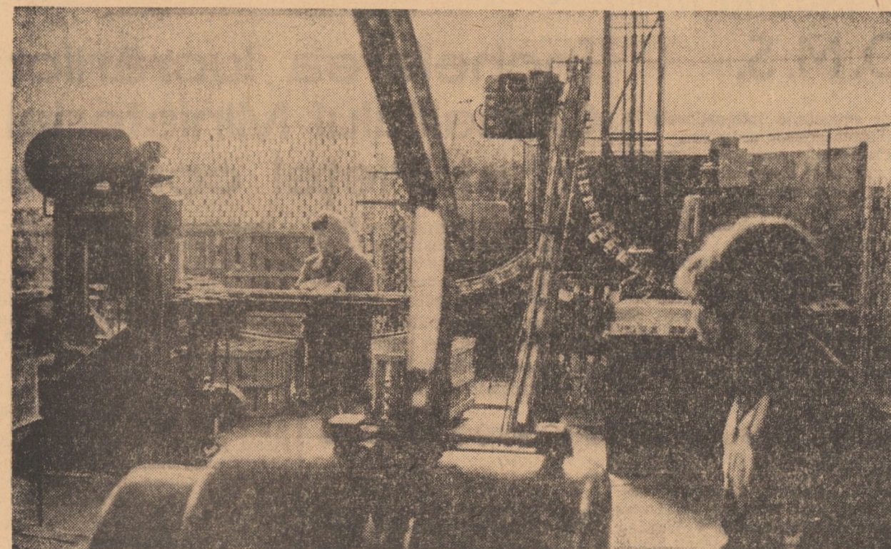
Linia automată de fabricat cutii pentru conserve a Fabricii de preparate și conserve de carne Sibiu, cu o capacitate de 100 cutii/minut
