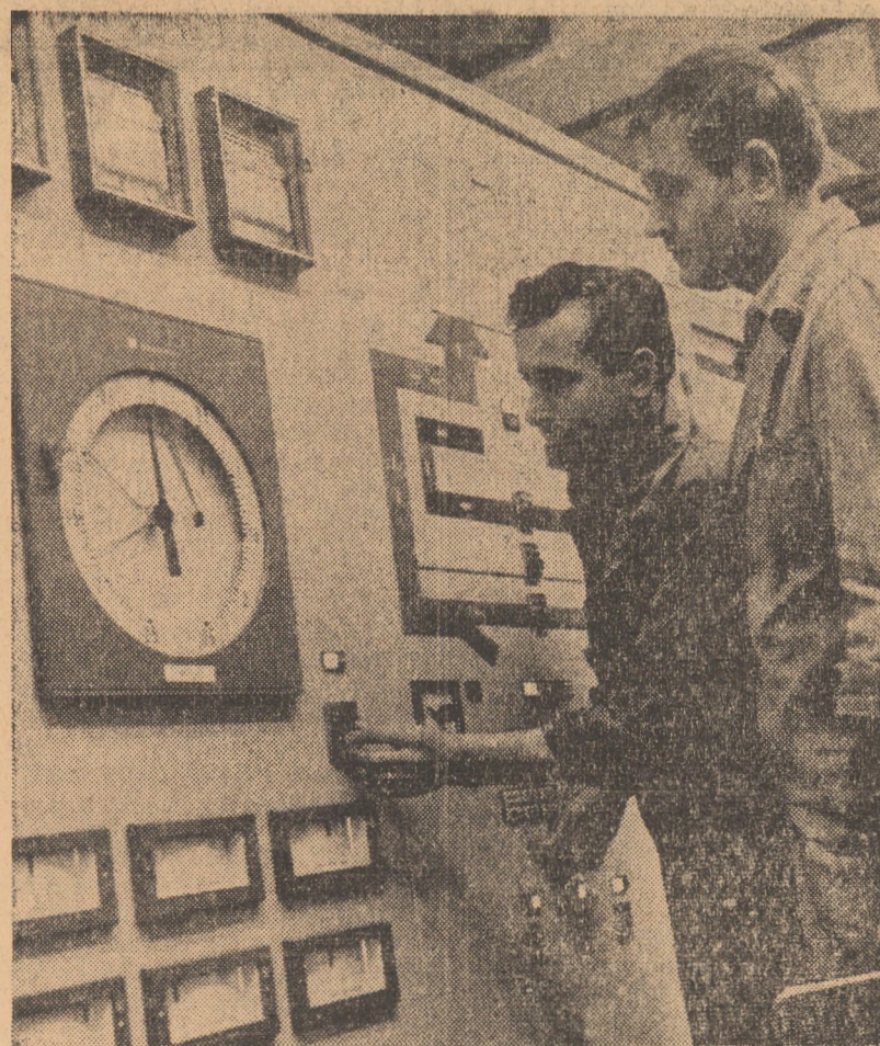
Noul cuplor automat de topit sticlă în întreprinderii „Vitrific” din Mediaș. În fotografie: cabina de comandă de unde se urmărește buna funcționare a cuplorului
