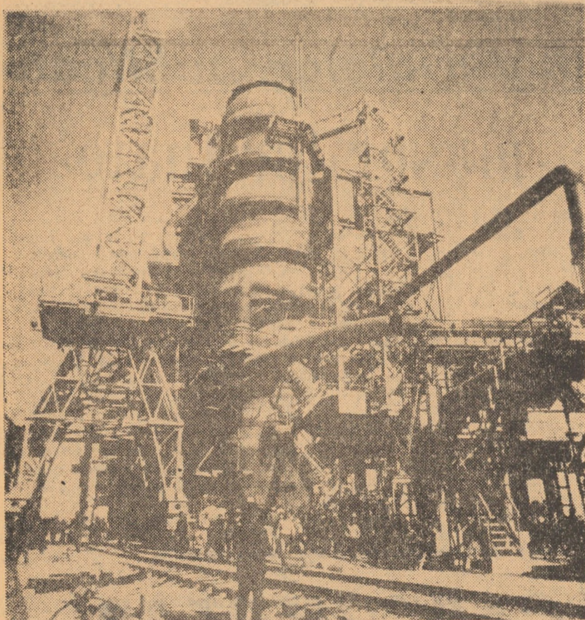
IRAN. Lucrările pe șantierul noului uzine metalurgice din Isfahan sunt într-o fază avansată. În foto: construcția primului furnal
