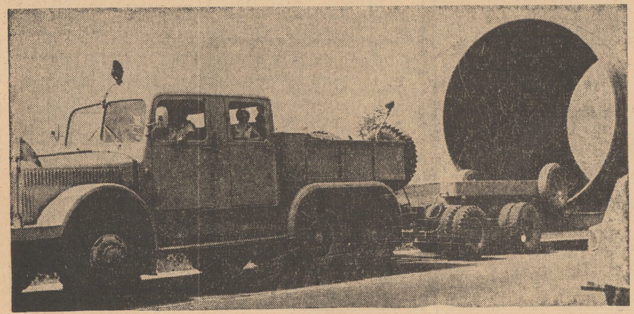
Un nou tronson este gata. El se adăugă altor zeci și zeci, produse de uzina „Independența”, pentru Hidrocentrula de pe Lotru. În clișeu: în timpul transportului uzina — hidrocentruală
