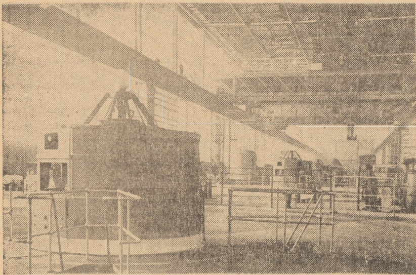
U.R.S.S. Ultimul agregat al celei mai mari hidrocentrale din lume, cea de la Krasnoïarsk, a intrat recent în funcțiune. Hidrocentrala va produce 5 milioane kW energie electrică. În fotografie: Sala mașinilor hidrocentralei
