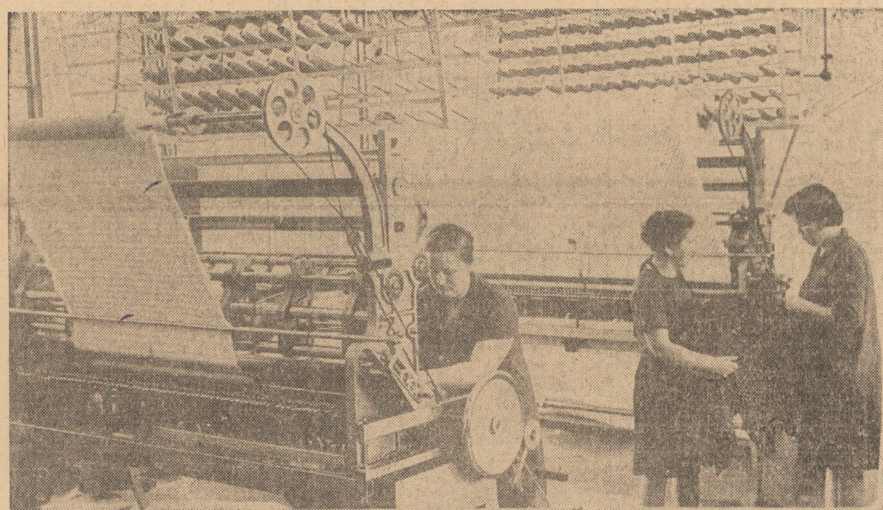
La cele două mașini de matlasat de la fabrica „Măteasa roșie” Cîsnădie, utilaje moderne de înaltă tehnicitate, unice în țară de acest tip, se obține într-o zi o producție de peste 1200 metri liniari de țesături pentru canadiene, pardesii, rochiile de casă etc.
