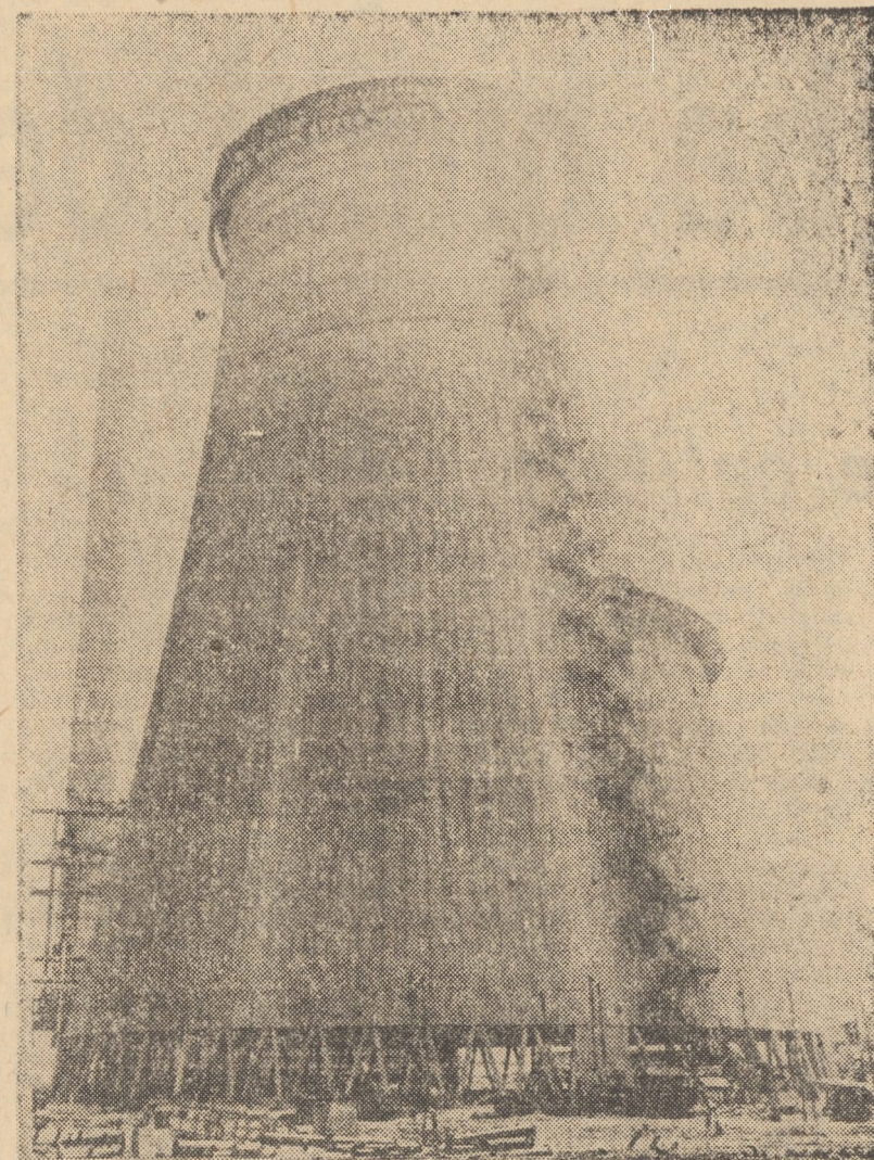
R.D.G. Termocentrala de la Boxberg, regiunea Cottbus va fi cea mai mare termocentrală din Europa centrală, cu o putere de 3 000 de megawați. Energia produsă aici ar putea alimenta două orașe de mărimea Leipzigului. Pentru sistemul de răcire al apei a fost nevoie de construirea mai multor stăvile. În fotografie: Turnul de răcire, primul gata la Boxberg, va începe să funcționeze în curînd
