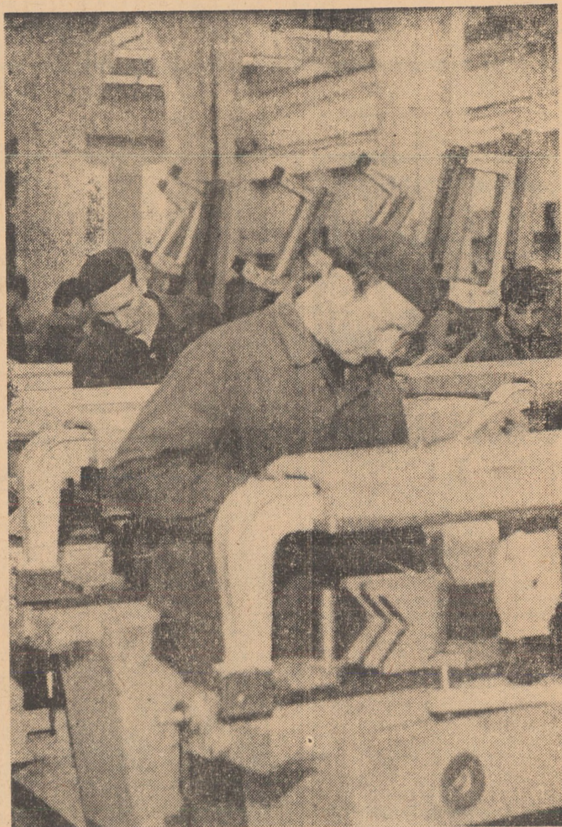
Uzina mecanică Sibiu. Se montează fierăstraie alternative, cunoscute și apreciate și peste hotarele țării
