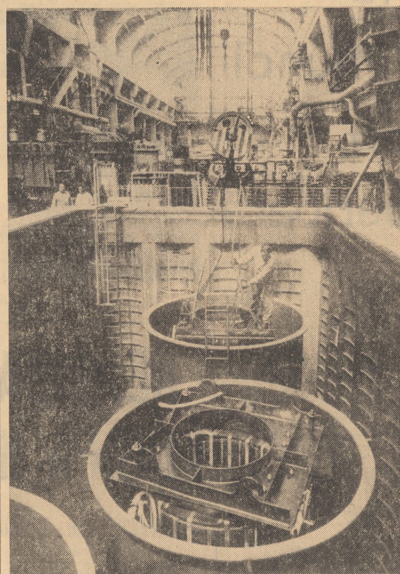
R.S. CEHOSLOVACĂ. Două transformatoare gigantice de trei faze fiecare cu o putere de 240 MVA și un voltaj de 242/15 kV, sint în fază de asamblare la fabrica de mașini electrice „Skoda”, din Doudlevec, lângă Plzen, destinate centralei electrice de la Brazi, Ploiești. Aceste transformatoare, cele mai mari care s-au produs până acum în fabrică, cântăresc fiecare 216 tone și au o lungime de 8 m, o lățime de 3,33 m și o înălțime de 4,8 m și vor fi livrate României în trimestrul trei al acestui an. În foto: bobinele sint ridicate din furnalul de vacuum la fabrica de mașini electrice „Skoda” din Doudlevec
