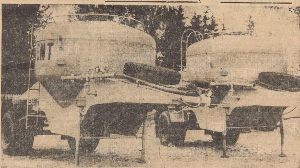
Printre produsele expuse în pavilionul E.R.E.N. '69 se numără și semiremorcă de 7,3 m c pentru transportul cimentului în vrac. Încă de atunci parametrii săi tehnico-funcționali au recomandat-o ca pe un produs ce permite o manipulare economică a materialelor de construcție
