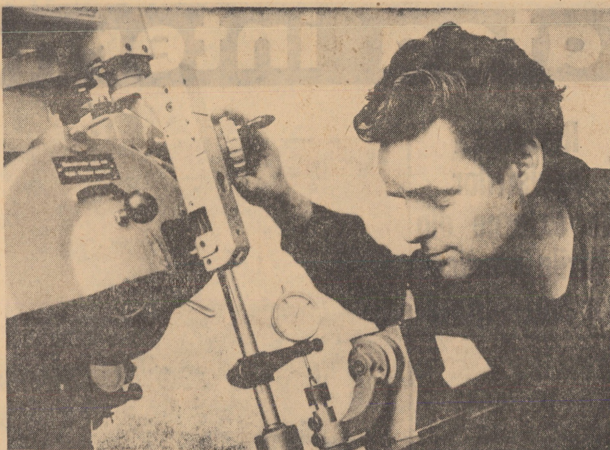
Locul de muncă al comunistului Petre Antobie este în atelierul scularie al uzinei „Balanta” Sibiu. Aici deservete o mașină de rectificat profile, utilaj de înaltă precizie, prelucrînd diferite dispozitive folosite la matrițe cu profile complexe. Avînd o vechime de 16 ani în meseria de rectificator, Petre Antobie reprezintă unul din mulțimea muncitorilor cu o bogată experiență profesională în munca lor de zi cu zi
