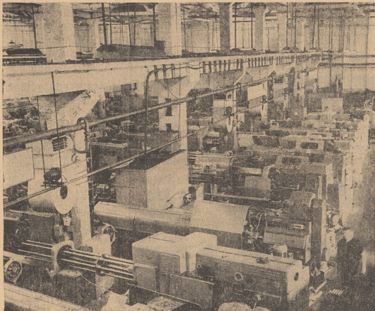
Linia de strunguri automate din secția mecanică III, atelierul lanț gall, al uzinei „Independența” Sibiu
