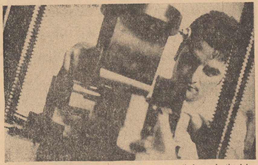
Uzina mecanică Mirza. La cererea diferitelor secții de producție, laboratorul uzinal efectuează probe de rezistență a materialelor la îndoire, rupere și elasticitatea sudurilor. Mostrele, în formă de eprubete, sînt supuse încercărilor la sudururile unor aparate speciale la care lucrează și laborantul Nicolae Hoadrea (fotografia noastră)
