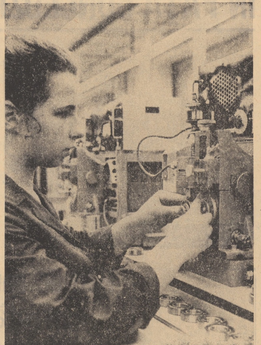
R.S. CEHOSLOVACA. Recent a intrat în probe o nouă linie pentru producerea rulmenților la fabrica „Bytčica ZVL” de lângă Zilina, în Slovacia Centrală. Linia, complet automatizată constă din 4 unități specializate fiecare pentru fabricarea unui tip de rulmenți. În foto: Linia de finisare a noii secții de rulmenți de la uzinele „Bytčica ZVL”, proiectată a produce anual 12 milioane rulmenți
