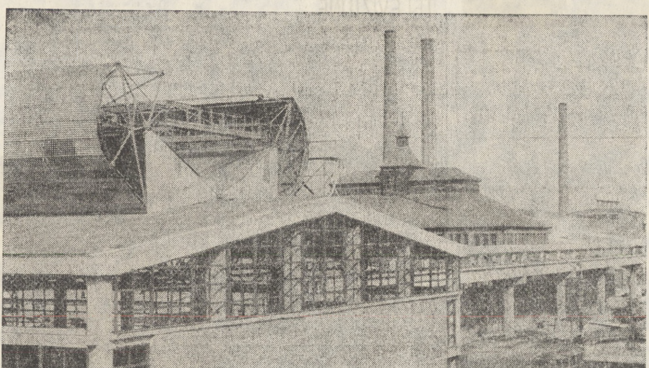
La Fabrica de geamuri din Mediaș se ridică noi hale de producție. În primul plan fotografie: hala cuptor, construită pe o suprafață de peste 1.350 m 2 , avînd o înălțime de 12 metri
