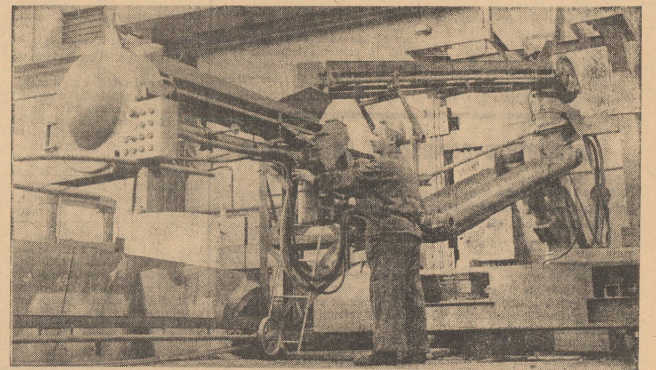
În turnătorile unor mari uzine metalurgice din țară sînt folosite utilaje moderne, de înaltă tehnică. Iată în fotografie mașina de format MP-61, unul dintre produsele uzinei „Independența” din Sibiu. Foto: HORST BUCHENNER
